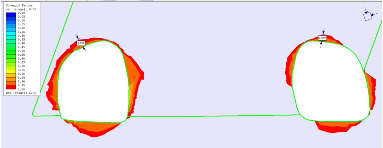
FIGURA 10 - Modelagem elástica da escavação com RS2
