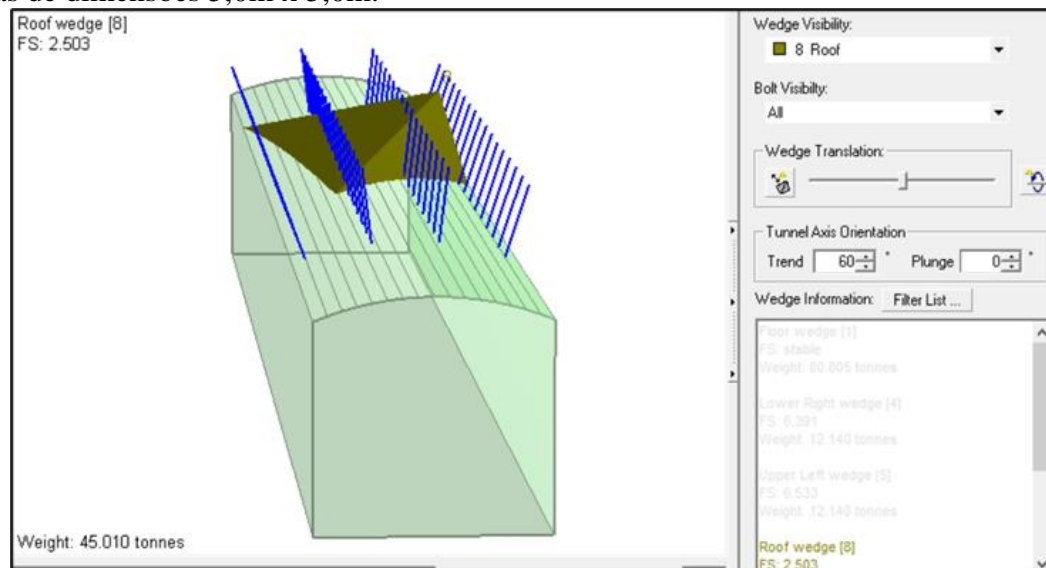
FIGURA 8 - Simulação feita no software Rocscience Unwedge com tirantes de 1,8 metros em galerias de dimensões 5,0m x 5,0m.
