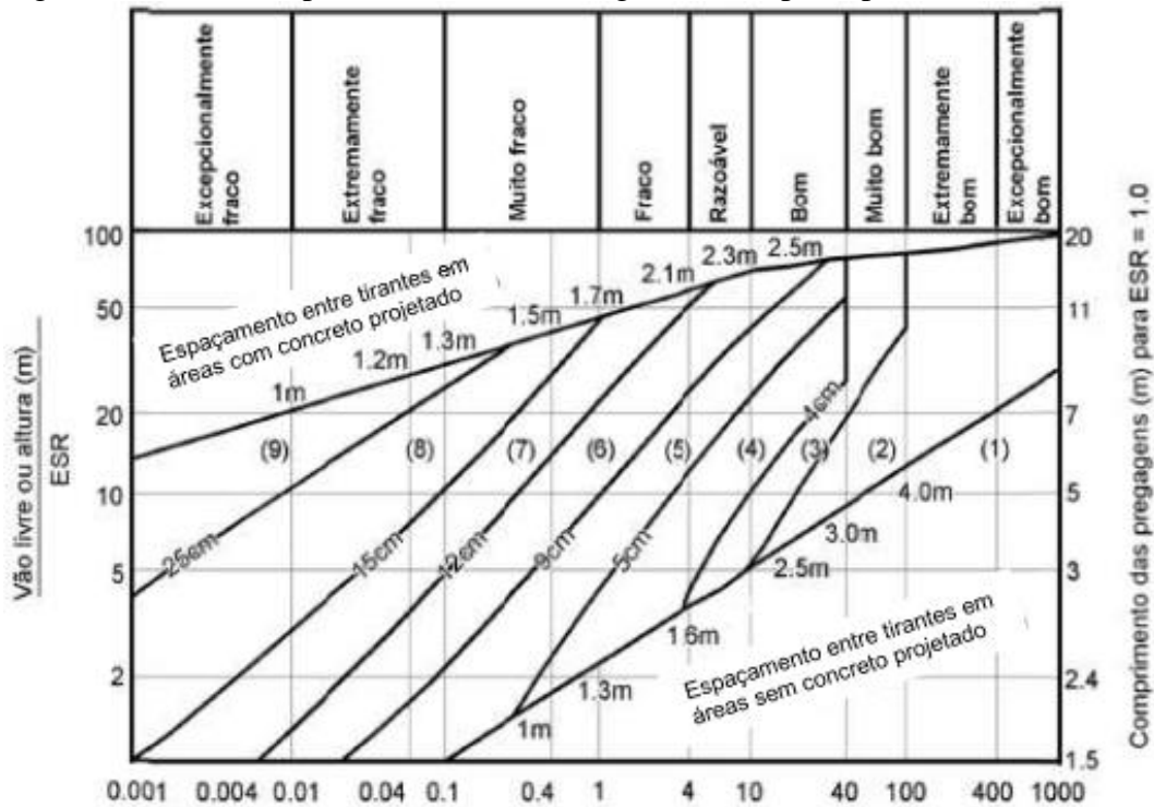
FIGURA 6 - Ábaco correlacionado a dimensão equivalente (DE), à qualidade do maciço segundo o sistema Q para se estimar as categorias de suporte permanente.
