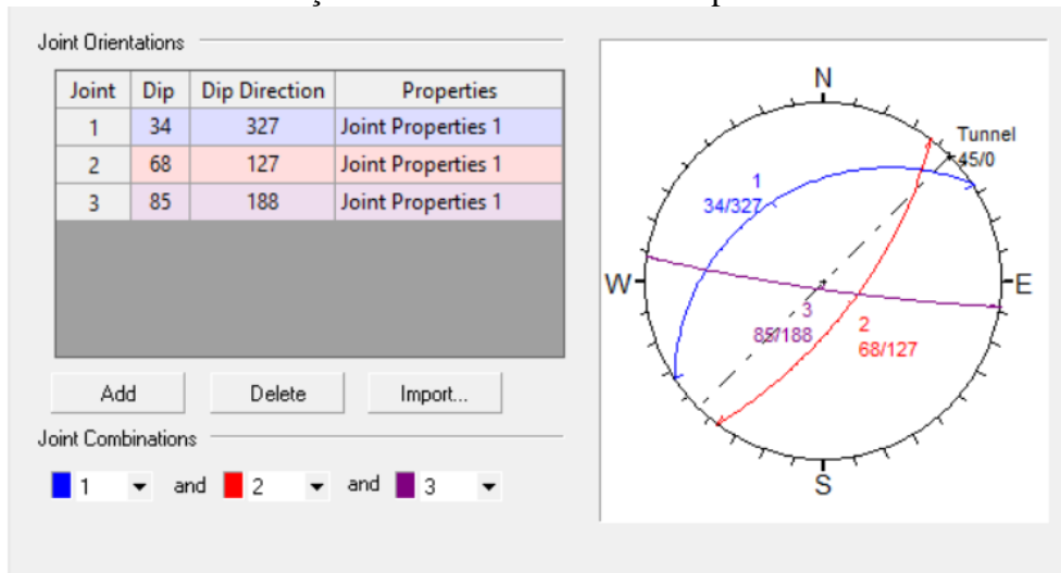
FIGURA 7 - Orientação das discontinuidades mapeadas na mina
