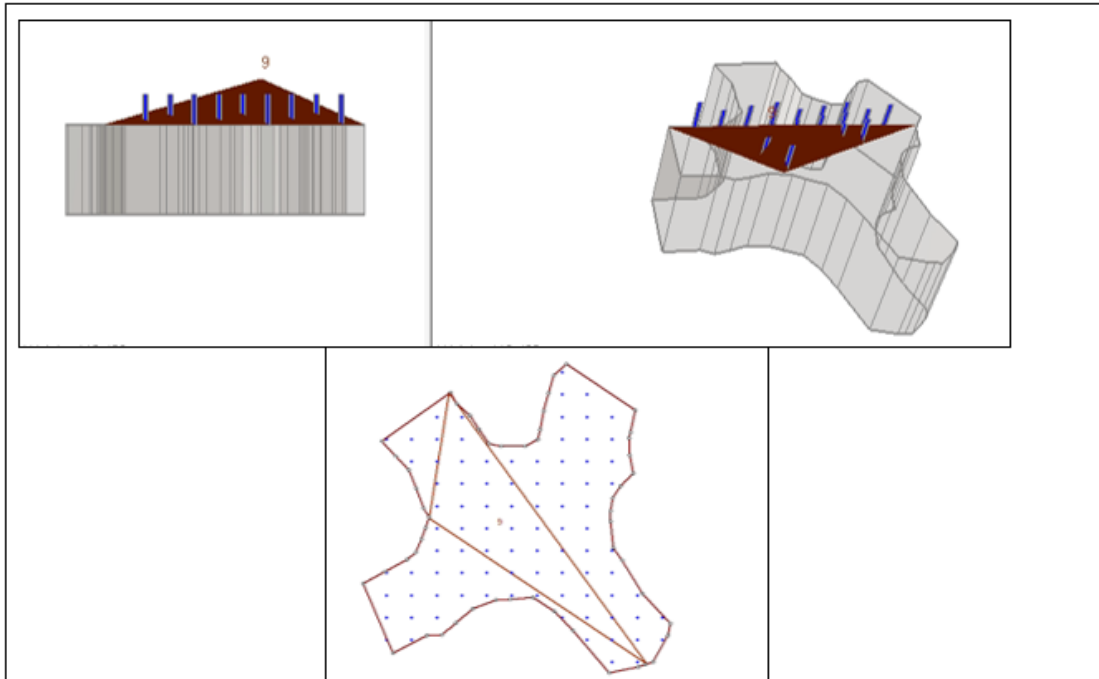
FIGURA 9 - Simulação da intersecção feita no software Rocscience Unwedge em galerias com vãos de 10 metros.
