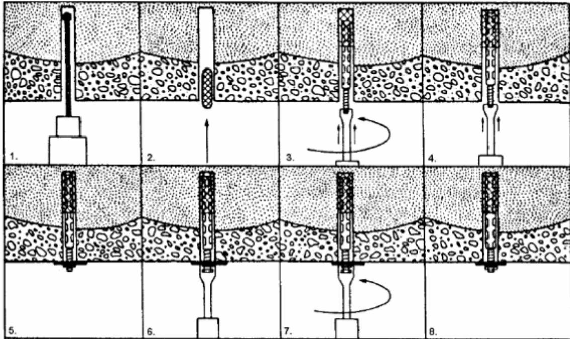
FIGURA 2 - Sequência de aplicação de tirantes com resinas.
