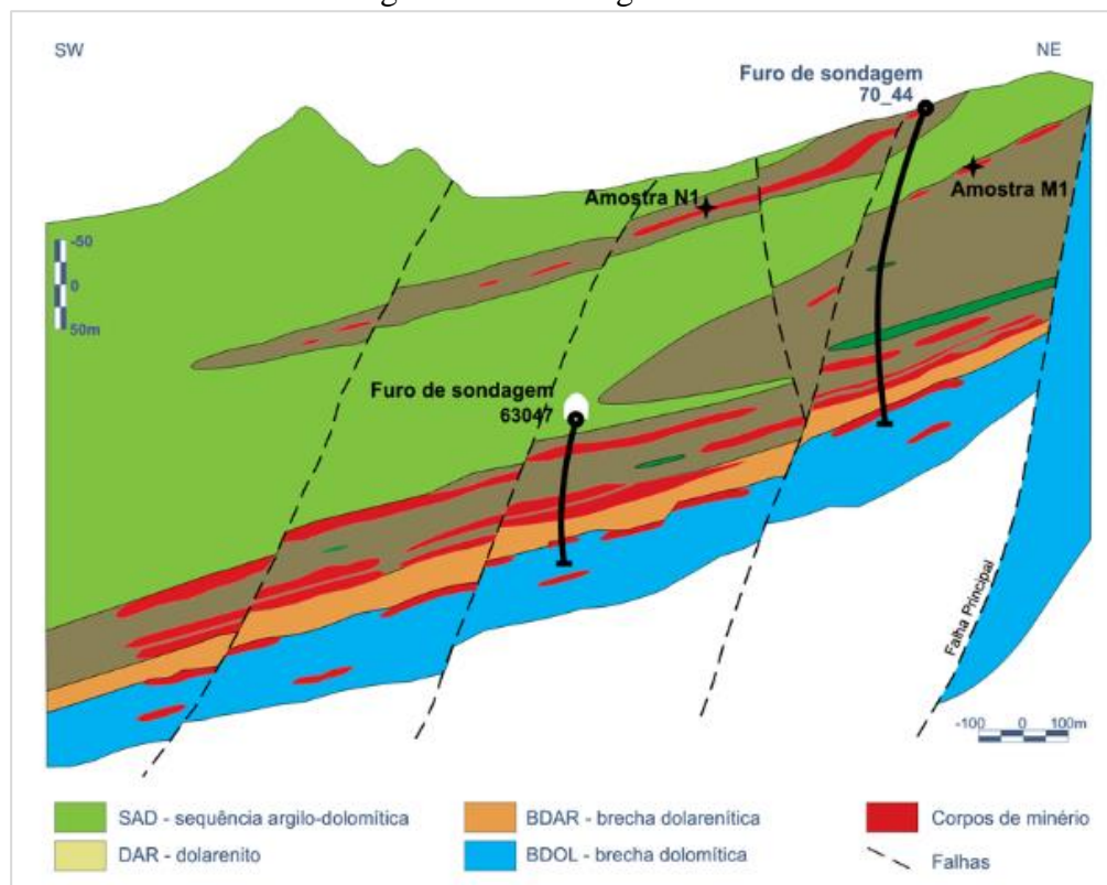
FIGURA 3 - Perfil Geológico de Morro Agudo
