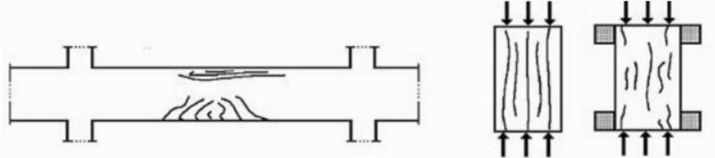
FIGURA 1 - Fissuras ocasionadas por cargas diretas
