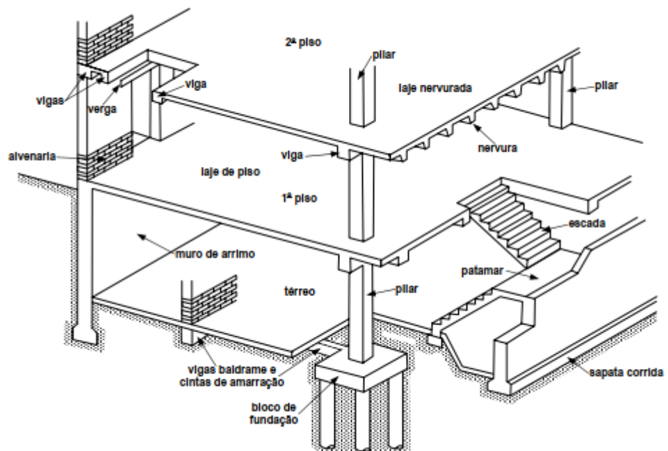
FIGURA 4 - Elementos Estruturais
