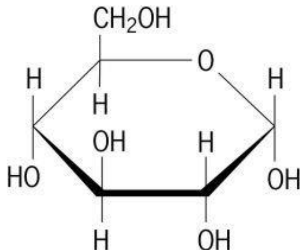
Figura 1- Estrutura química da glicose
